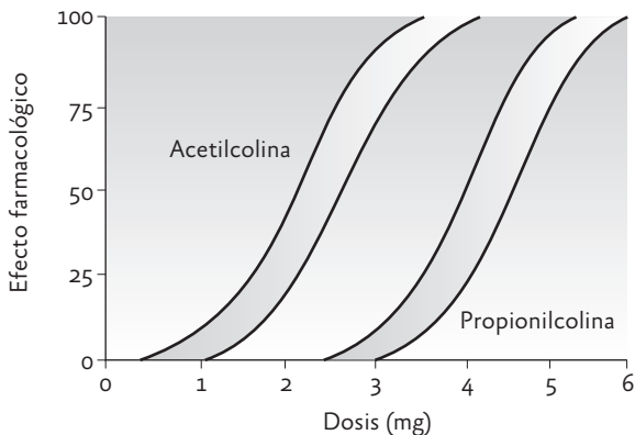
Figura 3-5. Afinidad.
