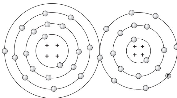
Figura 3-2. Unión iónica.
